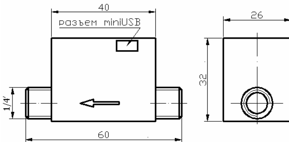
рис.1. Измеритель расхода газа
