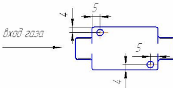
Рис.3. Крепление измерителя расхода газа.
